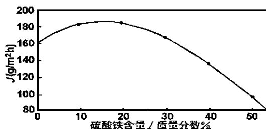
图 1 硫酸铁含量对 PVA/PSA 复合膜通量的影响
